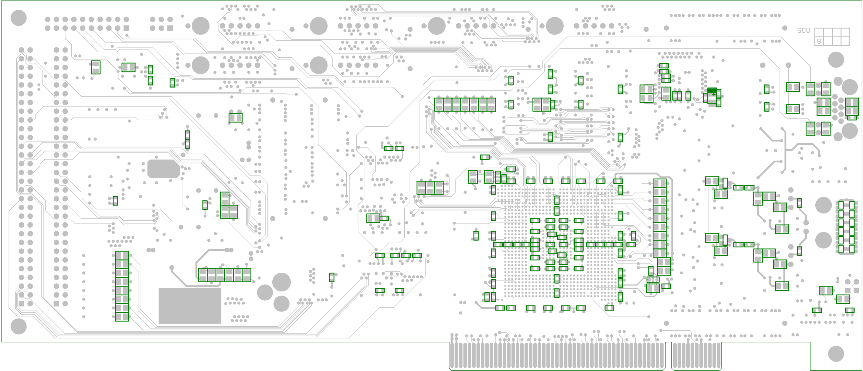
8 Couches Classe 5 Vias Traversantes
